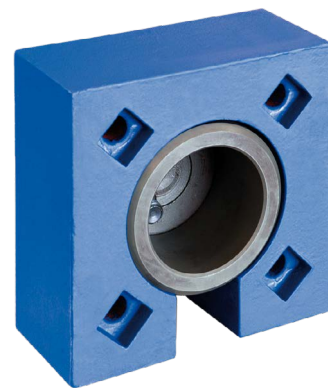
Wartungsfreier HEKO Lagerblock mit Lagerbuchsen
